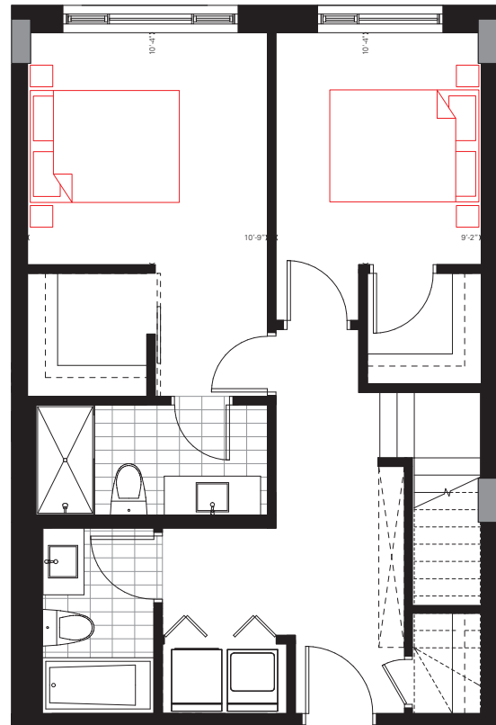
Étage 6 / Floor 6
